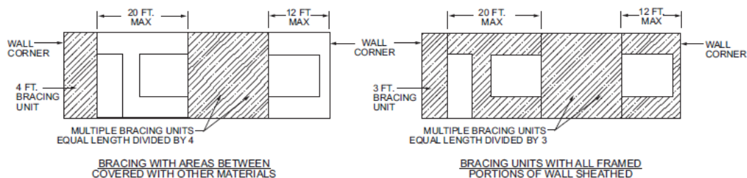
FIGURE 602.12.5
